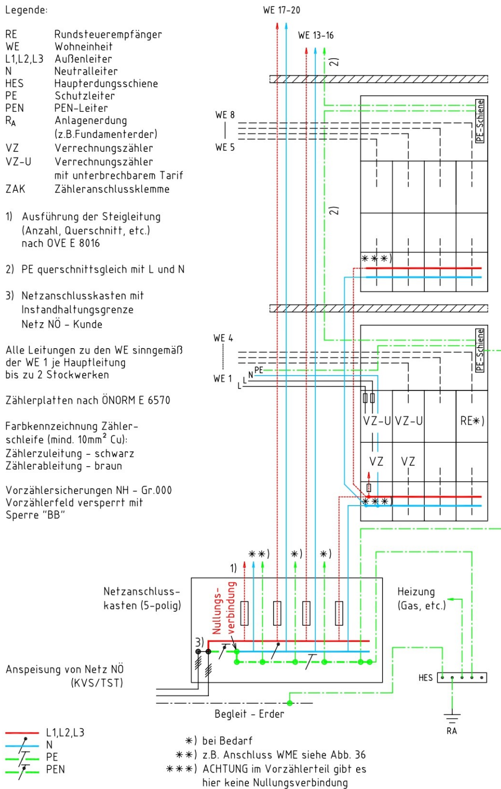
Abbildung 18: Schema für eine Wohnanlage mit Stockwerksverteilung für Direktmesseinrichtungen
